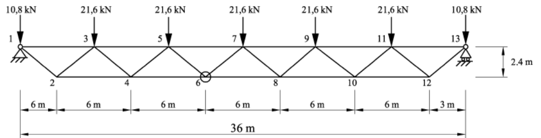
Bild 9.1: Ebener Fachwerkträger nach [2], Spannungsschwingbreite konstant
