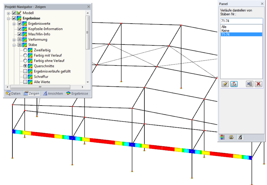
Bild 6.8: Stabfilter für Spannungsschwingbreiten eines Trägers
